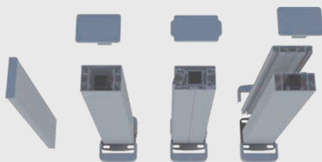
1/2 Poteau de départ 20 x 90 mm
