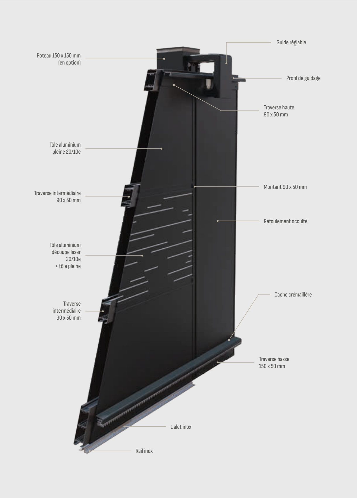
Guidage coulissant réglable à la couleur du portail
