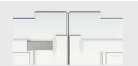
1 - Cadre inox soudé sur 4 faces recouvert d'un gainage blanc avec clé de gainage
